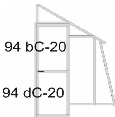
Prodloužené dveře o 20 cm
